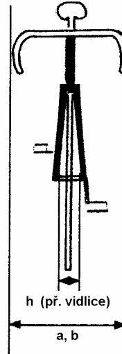
pohled zepředu
